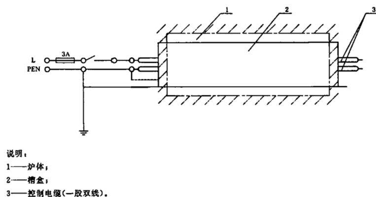
图 4 控制电缆接线
