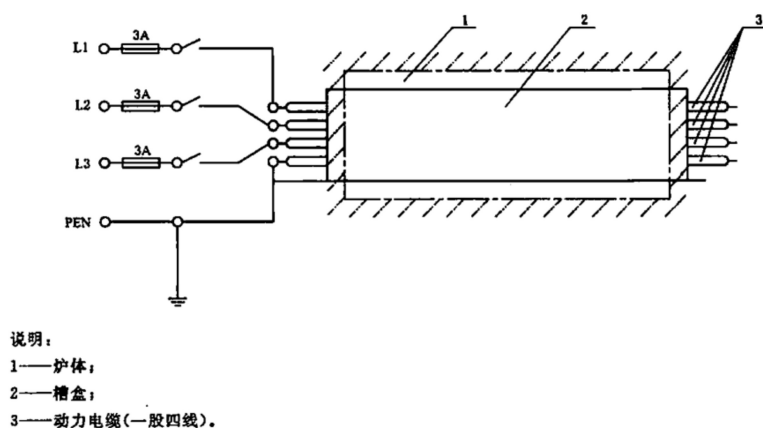
图 3 动力电缆接线
