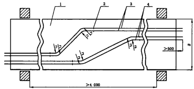
图1 槽盒在耐火试验炉内安装简图
