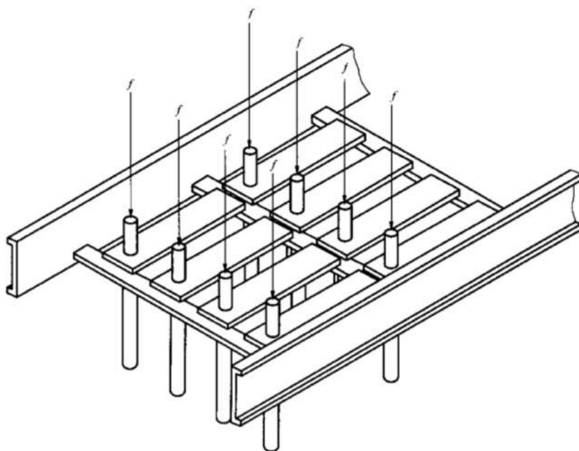
b) 终端三个横档上的载荷图
