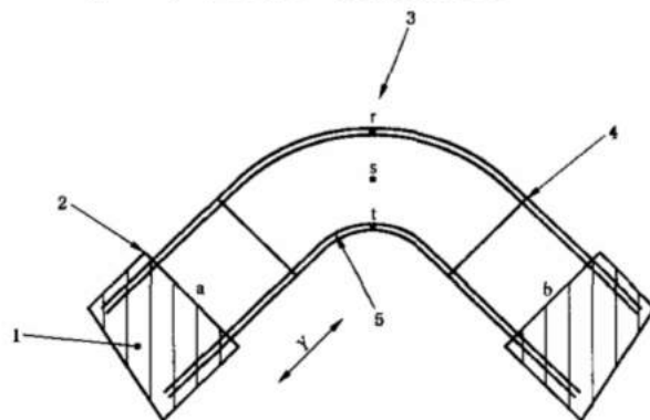
图4 单跨距安全工作载荷试验(见10.4)
