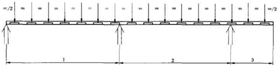
图 D.2 载荷加载块典型布置
