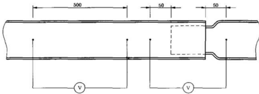
图 9 电气连续性试验
