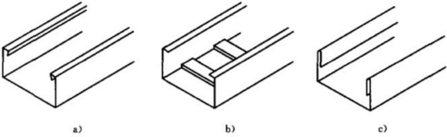
图 A.1 无孔电缆托盘直线段
