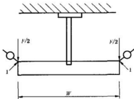
a) 天花板上的弯矩试验
