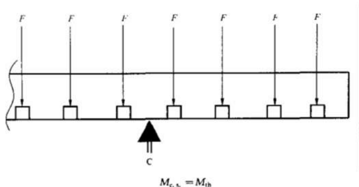
图 D.5 n 个横档
