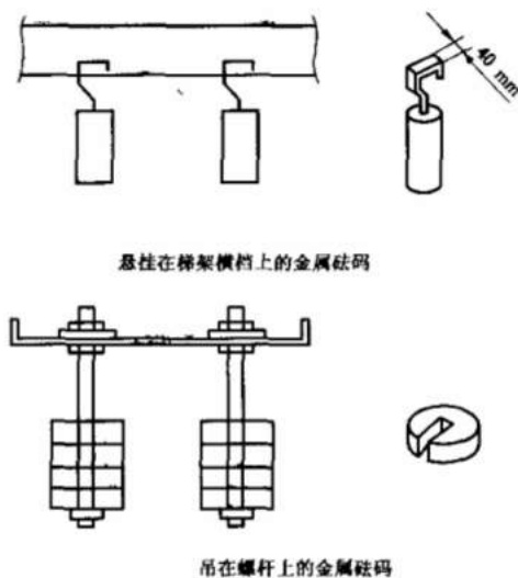
图 E.2 分别施加的点载荷
