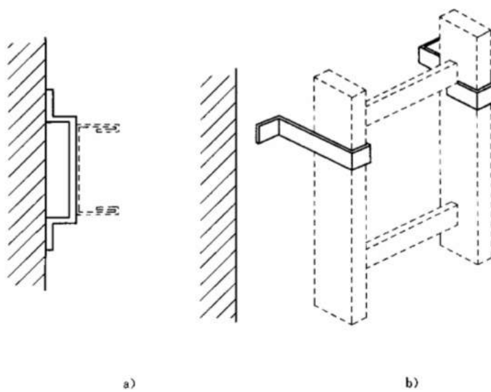
图 B.3 固定支架
