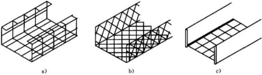
图 A.3 网状电缆托盘直线段
