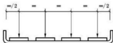
图 D.1 宽度范围内点载荷分布示例
