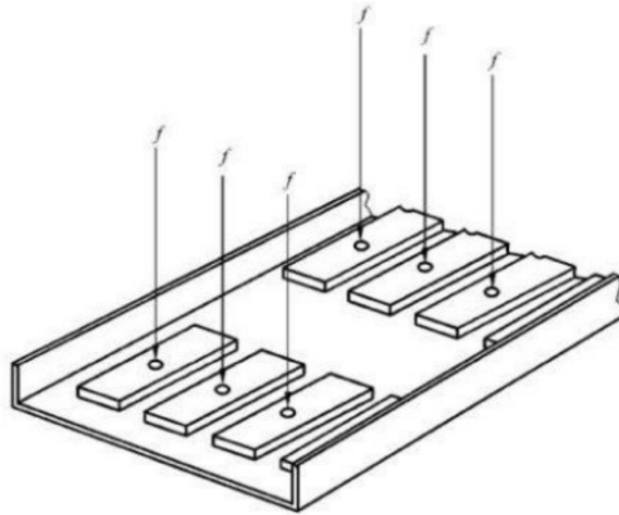
图 D.2 载荷加载块典型布置
