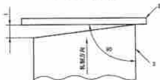
图3 镰刀弯的测量
