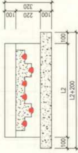
六根电缆直线槽
