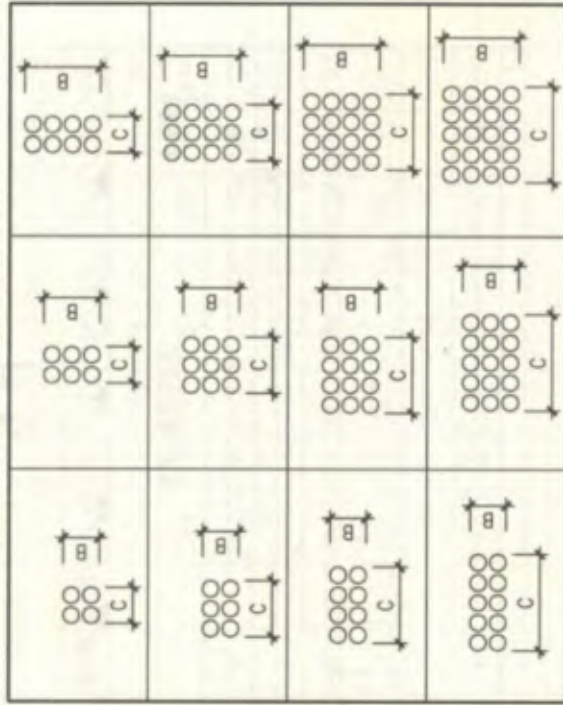
海泡石纤维水泥管常见组合方式
