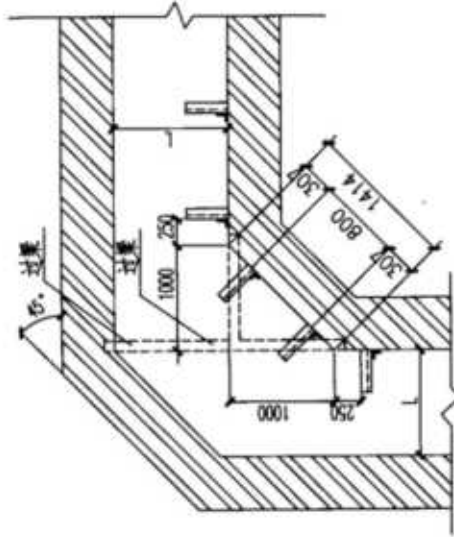
电缆沟转90° (二) (单侧支架)
