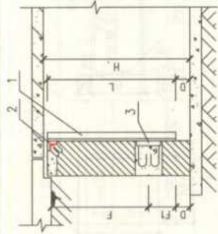
主架安装 (三)
