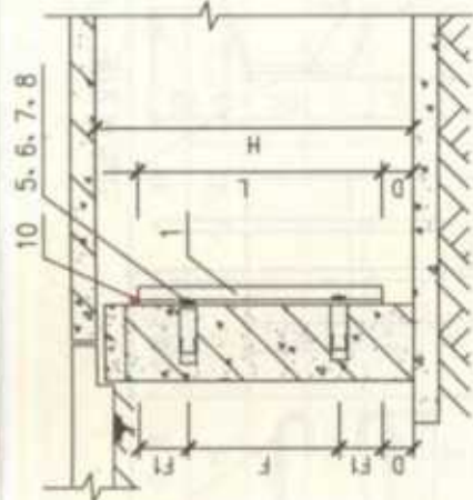
主架安装 (二)
