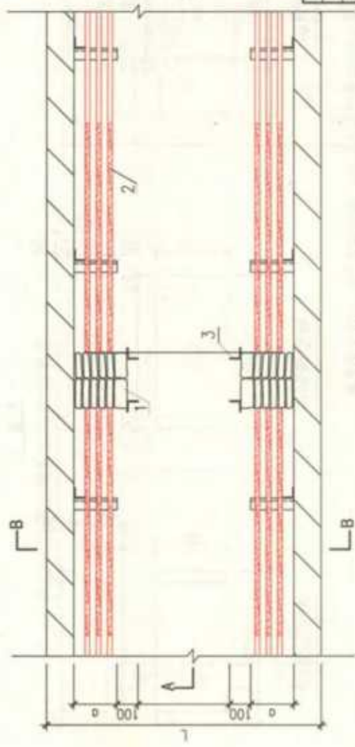
平面图
