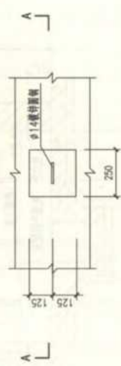
拉力环立面图
