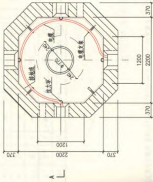
电缆在电缆井中预留平面图
