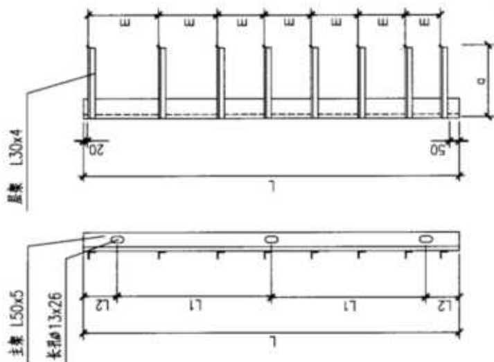
电缆支架
