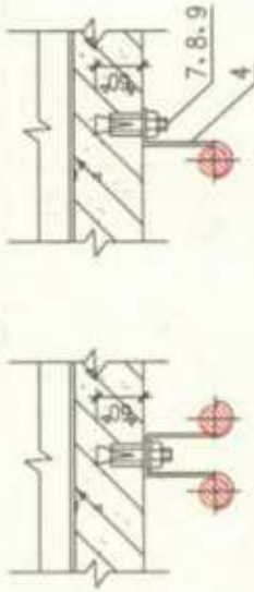
扁钢吊钩安装(一)
