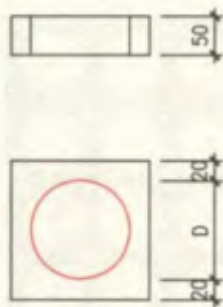
管枕
