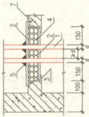
耐火隔板及矿棉封堵
