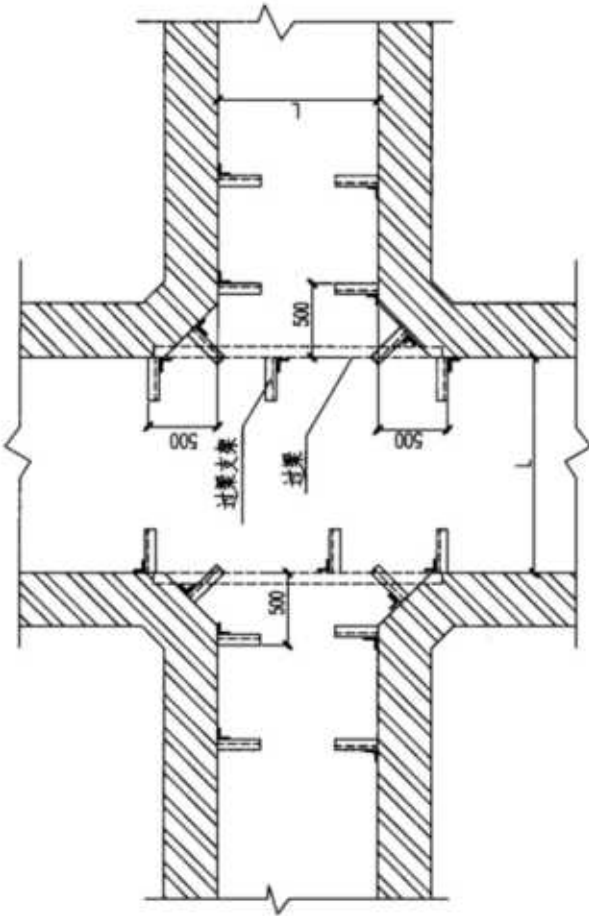
电缆沟交叉段
