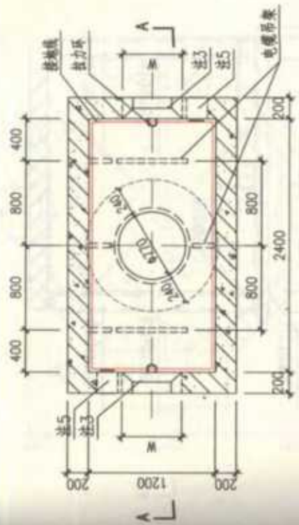
中型直通型电缆井平面图
