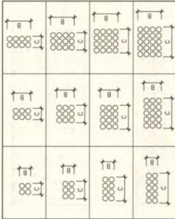
玻璃钢 (RPM) 电缆导管常见组合方式
