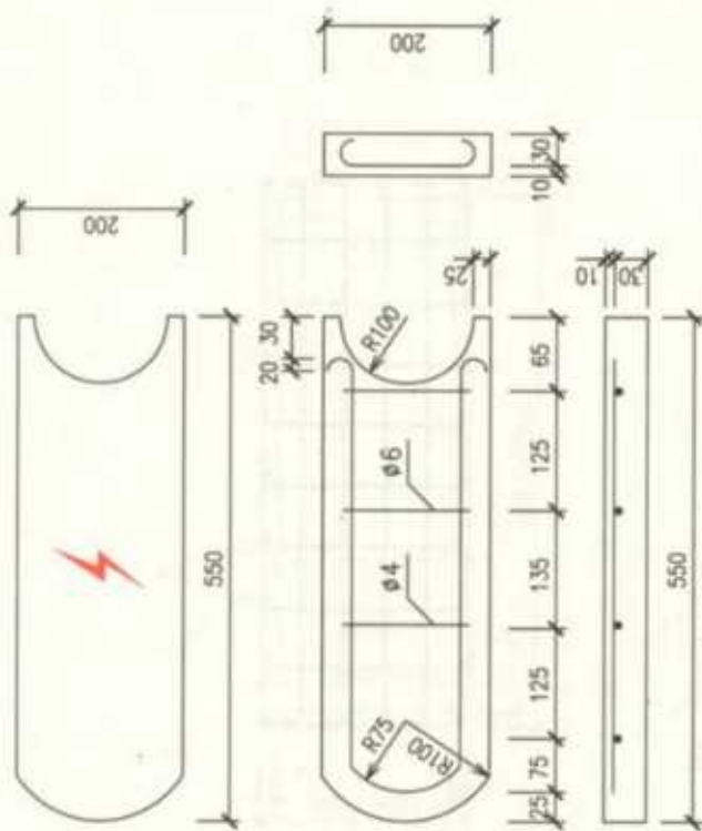
保护板(二)
