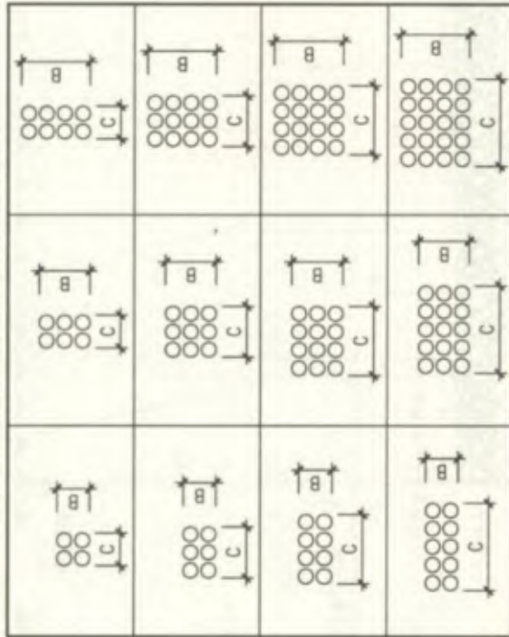
硬聚氯乙烯双壁波纹管常见组合方式
