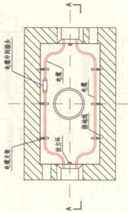
电缆在电缆井中中间接头平面图
