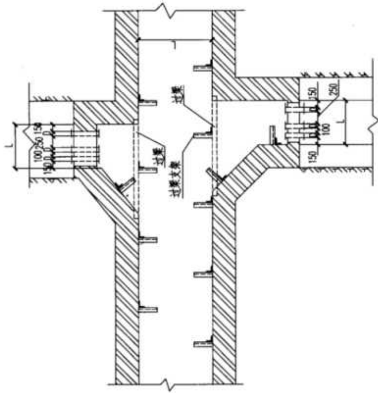
电缆沟分支段 (二)
