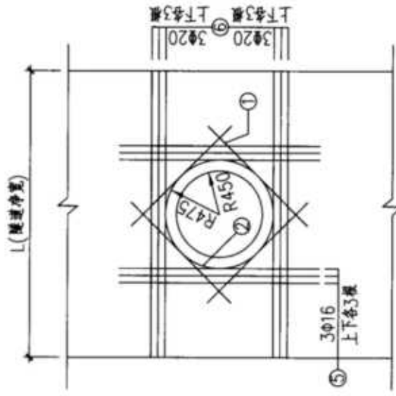
工作井口顶板配筋图
