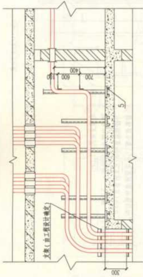
A-A
