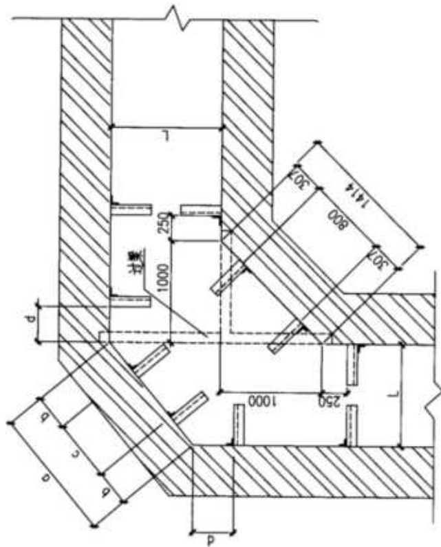
电缆沟转90° (双侧支架)
