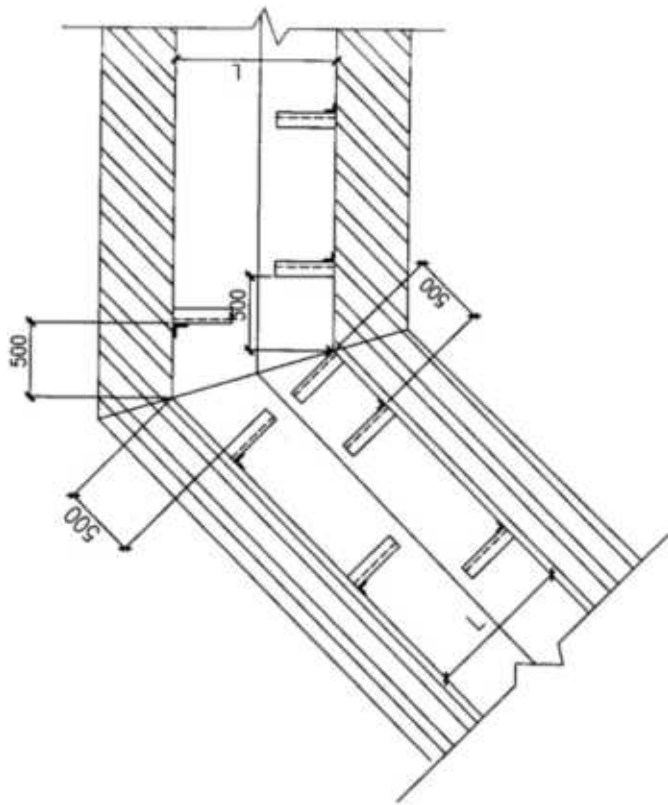
电缆沟转45° (双侧支架)
