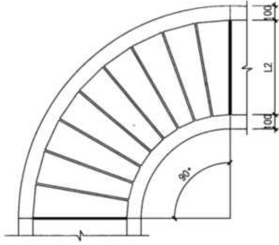
90° 转弯电缆槽安装 (需九个转弯槽)
