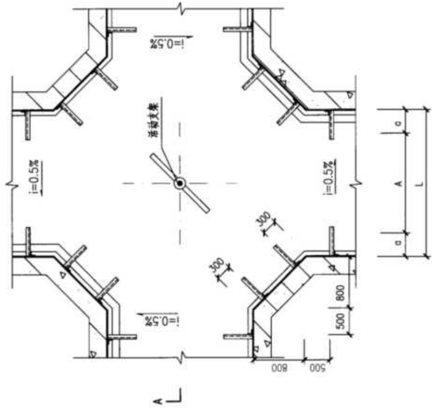
平面图
