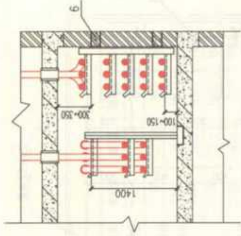
B-B
