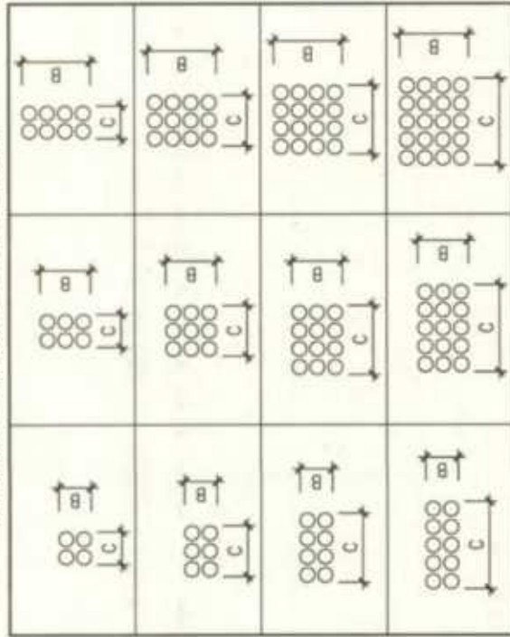
氯化聚氯乙烯电缆导管常见组合方式
