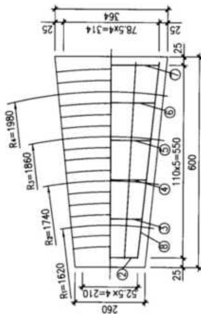
四根电缆转弯槽
