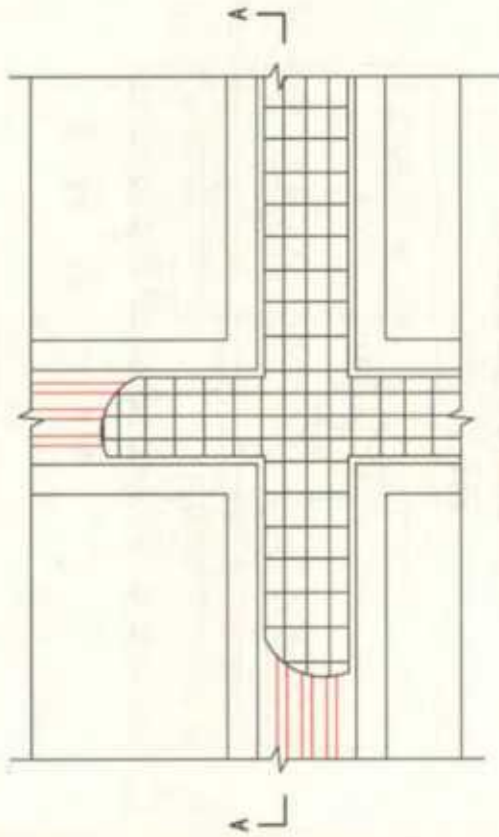
电缆与电缆交叉 (一)
