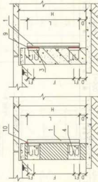
主架安装 (四)
