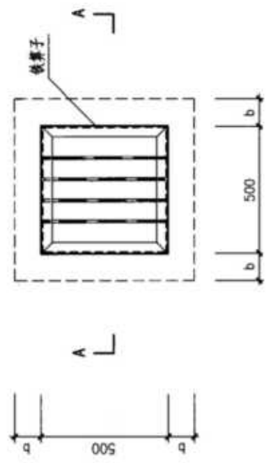
集水坑平面图
