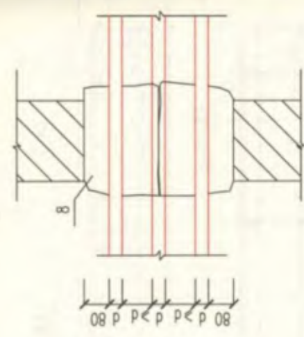
防火包封堵
