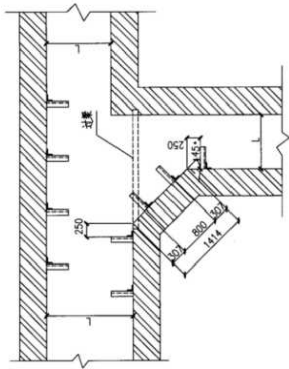
电缆沟分支段 (一)
