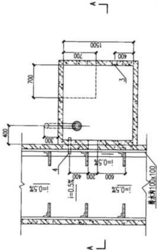
集水井平面
