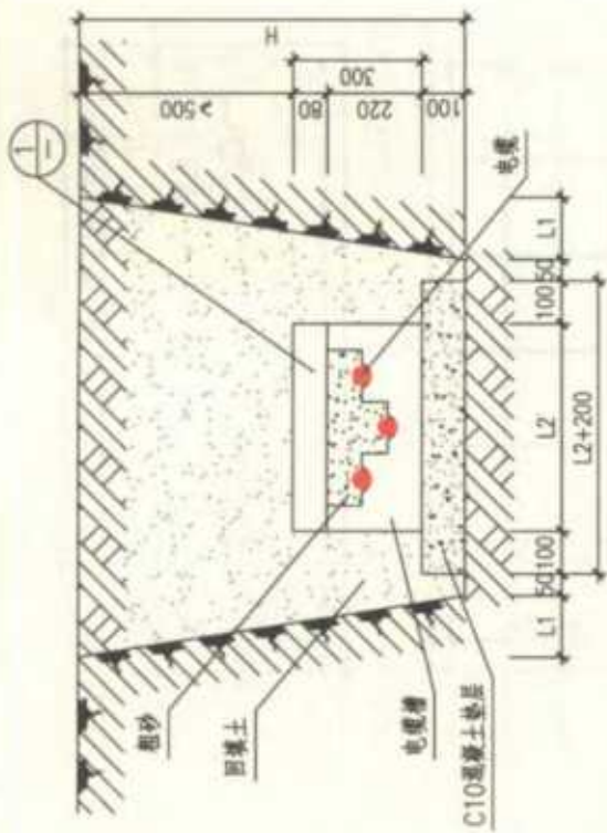
三根电缆直线槽
