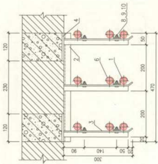
电缆在角钢支架上安装
