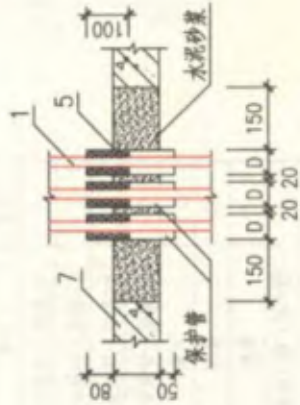
穿楼板保护管封堵
