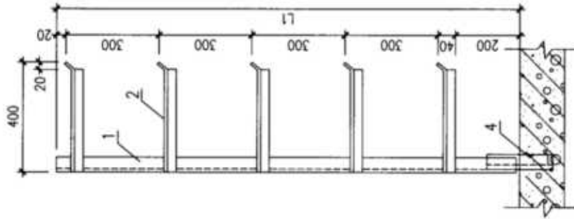
支架落地安装
