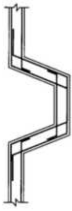
积水井配筋示意图
