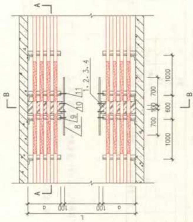
平面图
